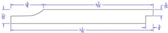
Fingerjoint - WC 105
