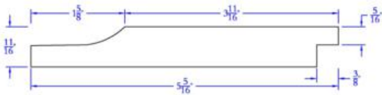
Fingerjoint - WC 105
